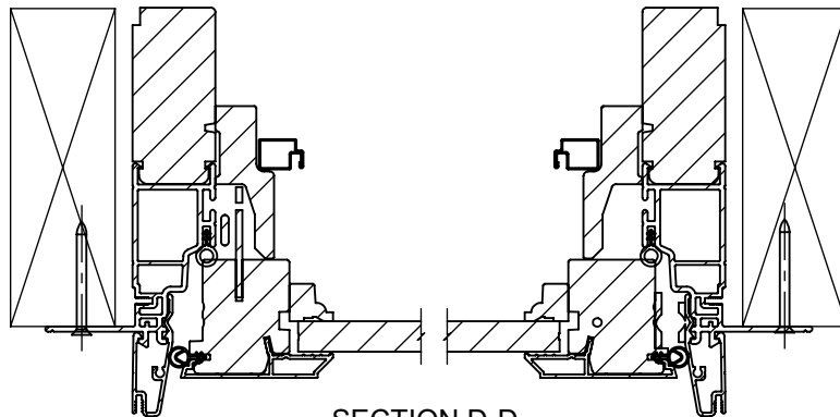
SECTION D-D SCALE 1 : 3
